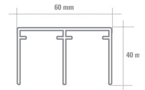
Top Guide (G22)
